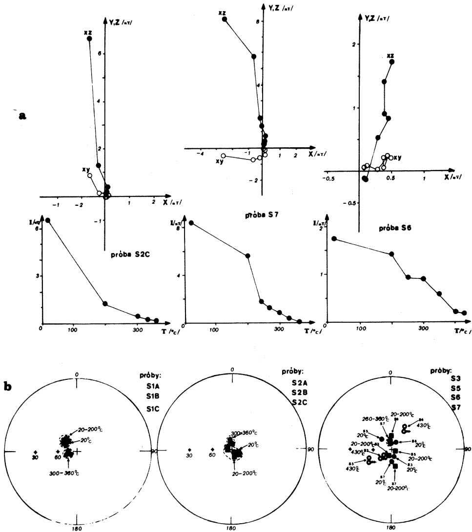
Fig. 5. Charakterystyka paleomagnetyczna szarych piaskowców droбноziarnistych kambru z otworu Sosnowiec IG 1
