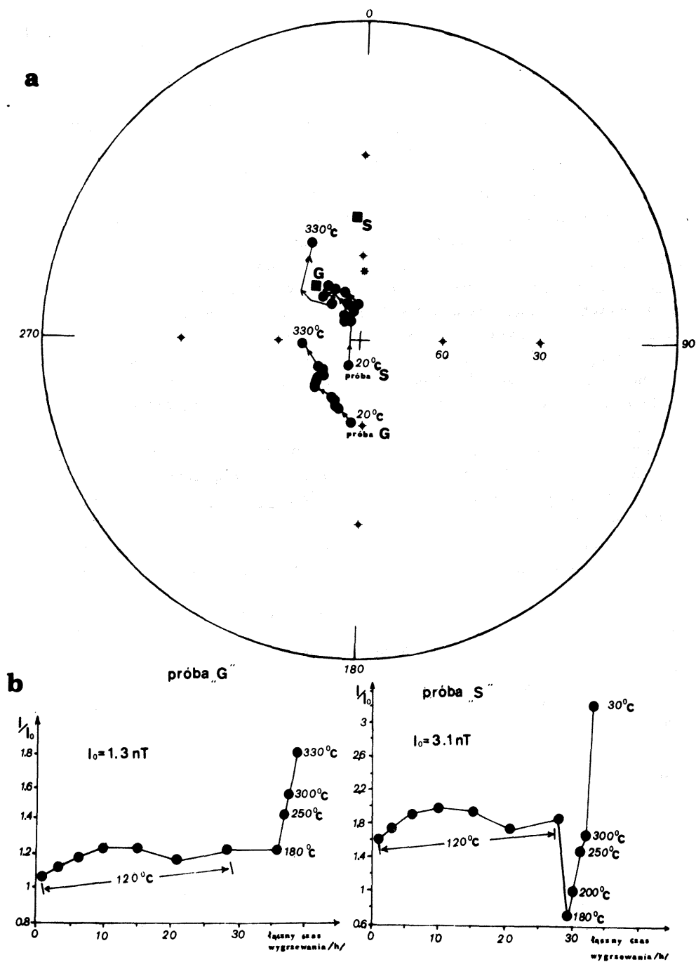
Fig. 3. Wyniki testu odtwarzającego proces utrwalania niskostabilnych składowych NRM w piaskowcach kambryjskich z otworów Goczałkowice IG 1 i Sosnowiec IG 1
