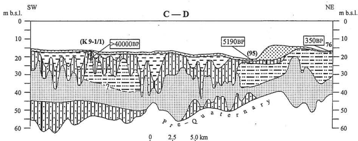
Fig. 3. Geologic cross-section C-D For explanations see Fig. 2 Przekrój geologiczny C-D Objaśnienia jak na fig. 2
