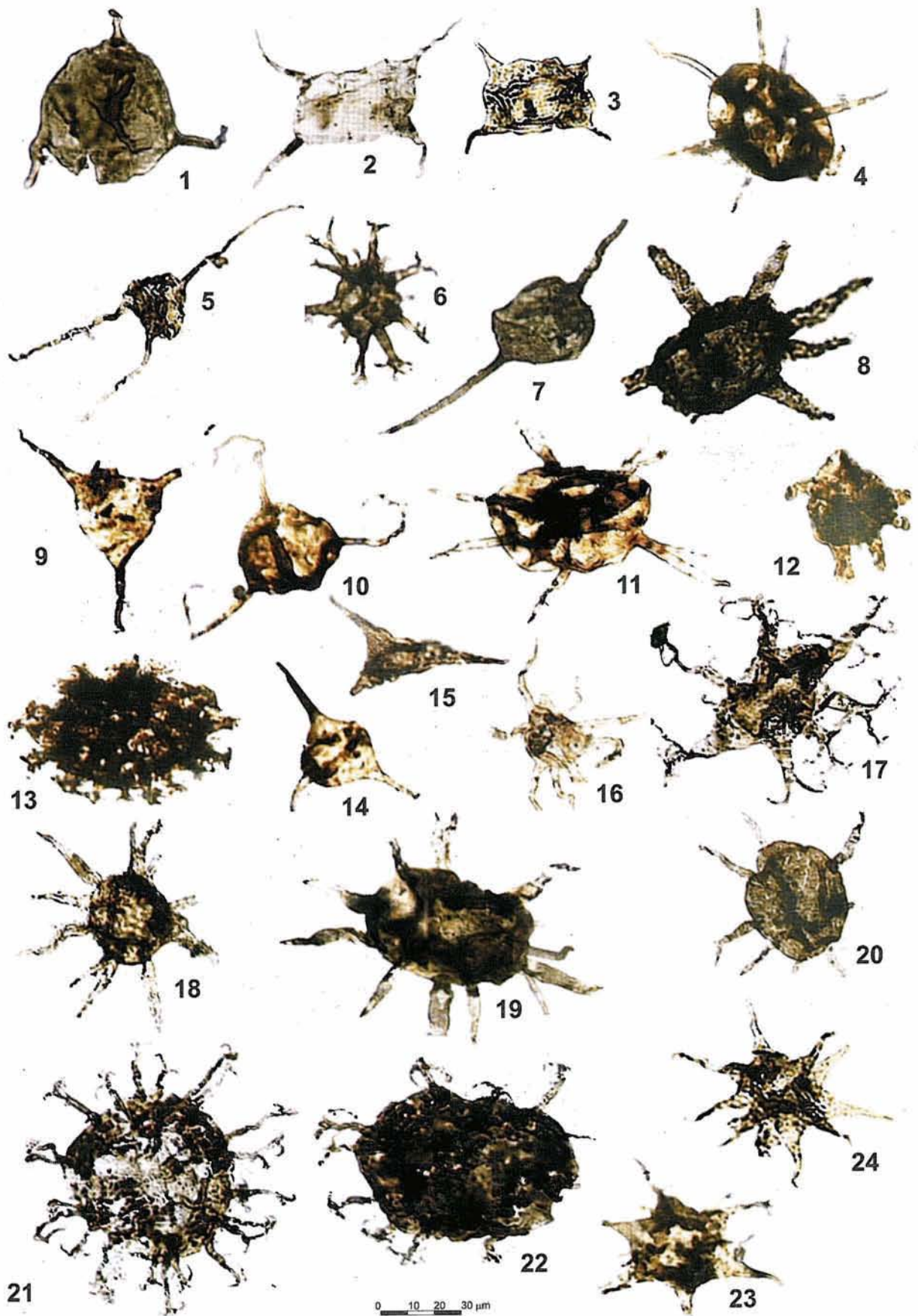
1. ? Veryhachium sp., 2404.0 m. 2, 3. Veryhachium lairdii (Defflandre): 2 — 2757.5 m, 3 — 2893.0 m. 4. Baltisphaeridium cf. longispinosum Eisenack, 2893.0 m. 5, 10, 14. Veryhachium sp., 2893.0 m. 6. Diexallophasis sp., 2893.0 m. 7. Acritarcha gen. et sp. ind., 2893.0 m; 8. Baltisphaeridium calicispinae Górka, 2893.0 m. 9. Veryhachium trispinosum (Eisenack), 2893.0 m. 11, 19. Baltisphaeridium lancettispinae Górka, 2757.5 m. 12. Petaloferidium sp., 2893.0 m. 13. Peteinosphaeridium sp., 2893.0 m. 15. Veryhachium reductum (Dcunff), 2893.0 m. 16. Aremoricanium sp., 2893.0 m. 17. Multiplicisphaeridium sp., 2893.0 m. 18. Baltisphaeridium cf. calicispinae Górka, 2757.5 m. 20. Baltisphaeridium plicatispinae Górka, 2893.0 m. 21, 22. Exculibranchium sp.: 21 — 2404.0 m, 22 — 2757.5 m. 23, 24. Polygonium gracile Vavrdová, 2893.0 m. Nowa Wieś I borhole
