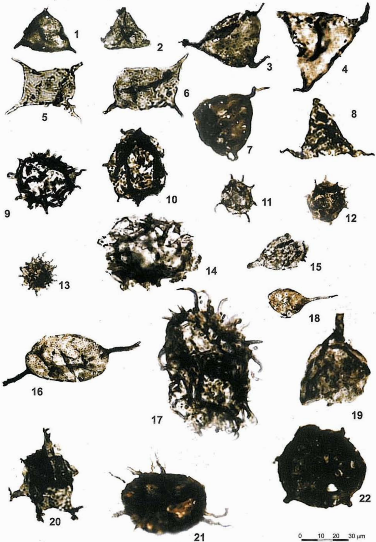
1, 3. Veryhachium trispinosum (Eisenack): 1 — 4713.0 m, 3 — 4715.0 m. 2, 4. Veryhachium reductum (Deunff): 2 — 4782.0 m, 4 — 4715.0 m. 5, 6. Veryhachium cf. lairdii (Deflandre): 5 — 4725.0 m, 6 — 5043.0 m. 7. Veryhachium cf. hamii Loeblich, 4725.0 m. 8. Veryhachium trispinosum ssp. geometricum Deflandre, 5000.0 m. 9, 10, 14. Polygonium sp. 1: 9 — 4715.0 m, 10 — 5043.0 m, 14 — 4715.0 m. 11, 12. Polygonium sp.: 11 — 4713.0 m, 12 — 4725.0 m. 13. ? Polygonium sp., 4725.0 m. 15, 19. Pirea sp.: 15 — 4715.0 m, 19 — 5000.0 m. 16. ? Orthosphaeridium sp., 4713.0 m. 17. Acanthodiacrodium sp., 4725.0 m. 18. ? Veryhachium sp., 4782.0 m. 20. Tylotopalla sp., 5000.0 m. 21. Baltisphaeridium cf. plicatispinae Górká, 4725.0 m. 22. ? Baltisphaera sp., 5043.0 m. Chojnice 5 borehole
