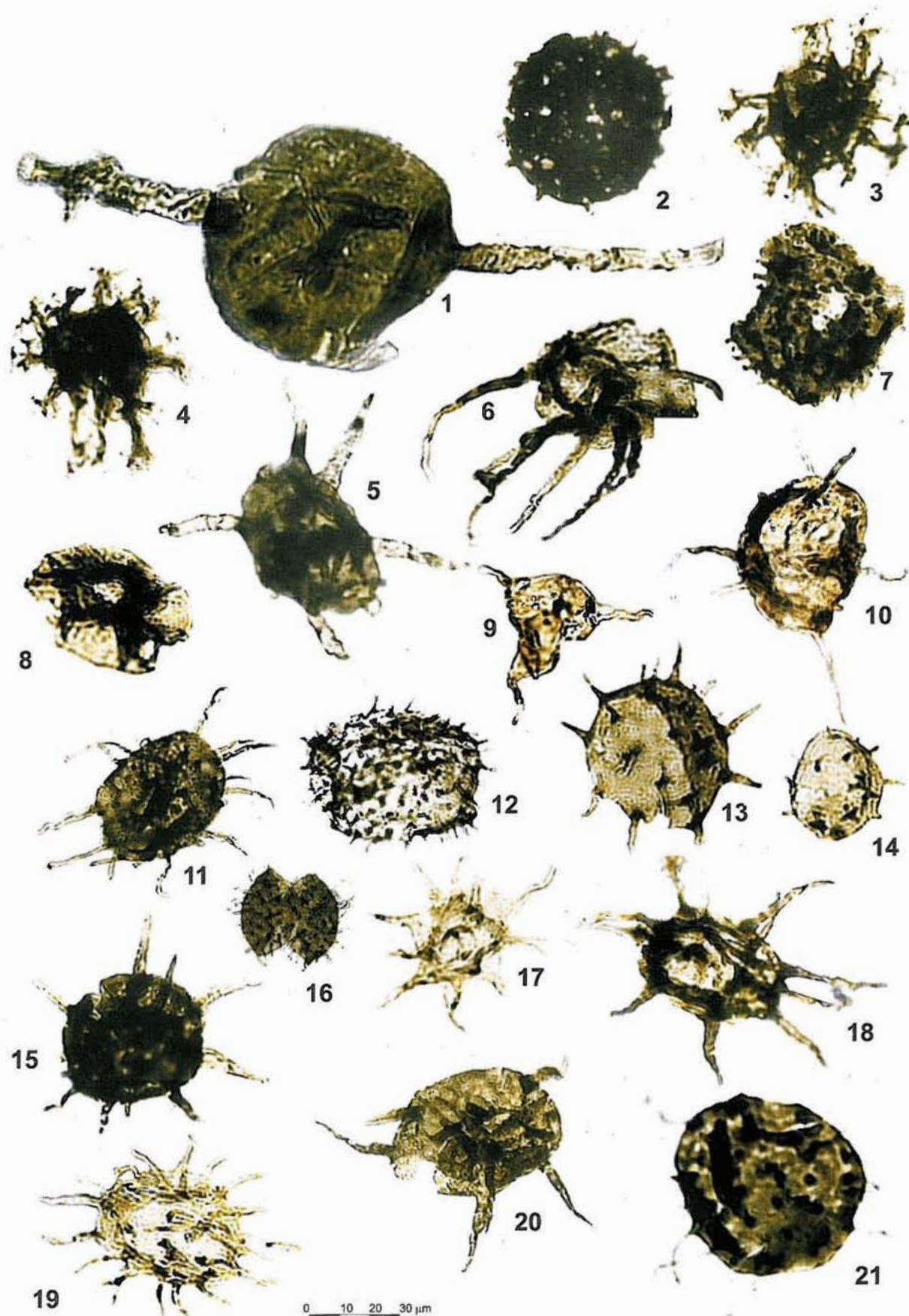
1, 5. Baltisphaeridium plicatispinae Górka, 3276.0 m, Ashgill. 2. ? Baltisphaeridium sp., 4423.5 m, Arcnig. 3, 4. Petinosphaeridium bergstromi Staplin, Jansonius et Pocock, 3114.8 m, Llanvirn. 6. Aremoricanium sp., 3114.8 m, Llanvirn. 7. ? Coryphidium sp., 3114.8 m, Llanvirn. 8. Cymatiosphaera sp., 3114.8 m, Llanvirn. 9. Veryhachium trispinosum (Eisenack), 3090.5 m, Ashgill. 10. Baltisphaeridium longispinosum Eisenack, 3090.5 m, Ashgill. 11. Baltisphaeridium cf. vieslavi Górka, 3114.8 m, Llanvirn. 12. Baltisphaeridium hamatum (Downic), 3114.8 m, Llanvirn. 13. Baltisphaeridium hirsutoides (Eisenack), 3114.8 m, Llanvirn. 14. Baltisphaeridium cf. hirsutoides (Eisenack), 3114.8 m, Llanvirn. 15, 20. Baltisphaeridium sp., 3114.8 m, Llanvirn. 16. Baltisphaeridium multipilosum (Eisenack), 3114.8 m, Llanvirn. 17. Polygonium gracile Vavrdová, 3114.8 m, Llanvirn. 18, 19. Polygonium sp., 3114.8 m, Llanvirn. 21. Acritarcha gen. et sp. ind., 3114.8 m. 1, 5 — Lębork IG I borehole, 2 — Kościerzyna IG I borehole, 3, 4, 6–21 — Gdańsk IG I borehole
